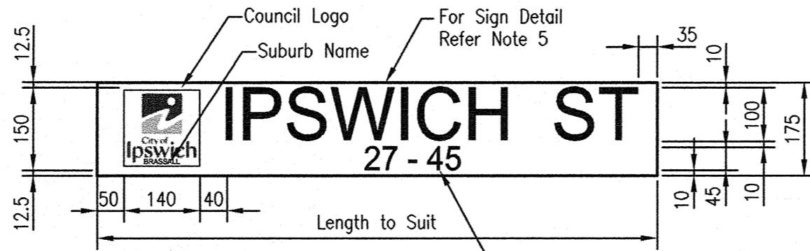
ICC SIGN PLATE DETAIL N.T.S.
