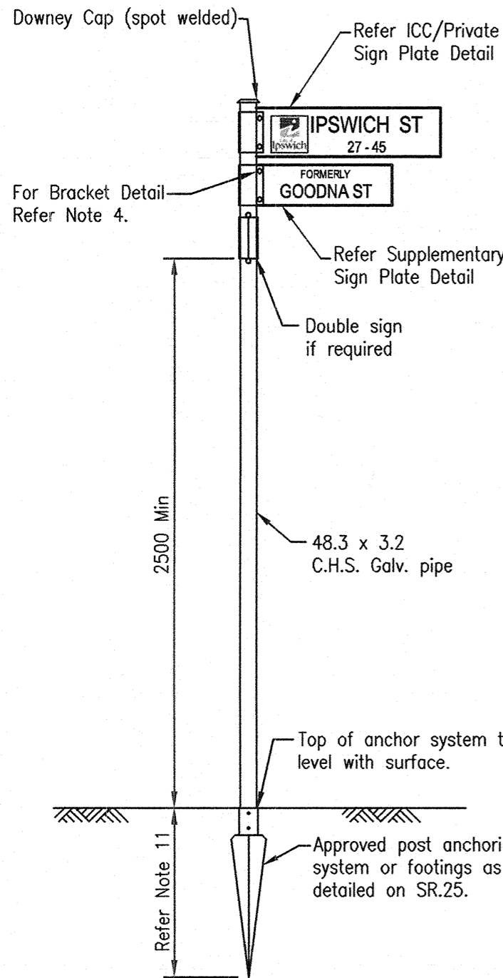
STREET NAME SIGN N.T.S.
