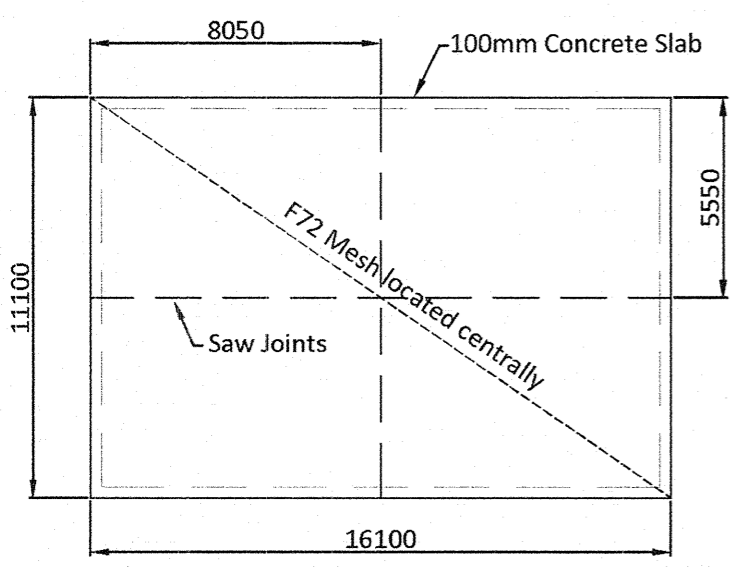
PLAN: SET OUT SCALE: 1:200
