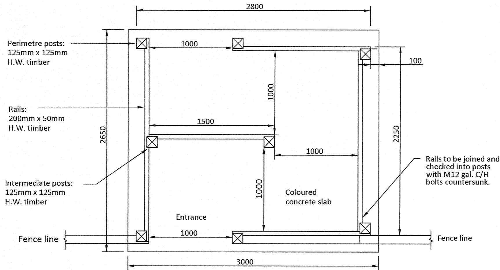
PLAN Scale: 1:25
